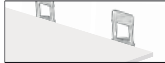
Posiziona due o più "Clip Fuga" al di sotto della piastrella. Posiziona una seconda piastrella.
